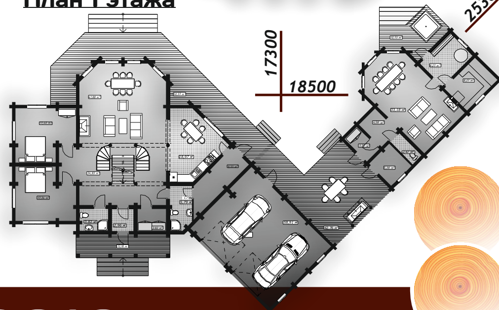
План 1 этажа
