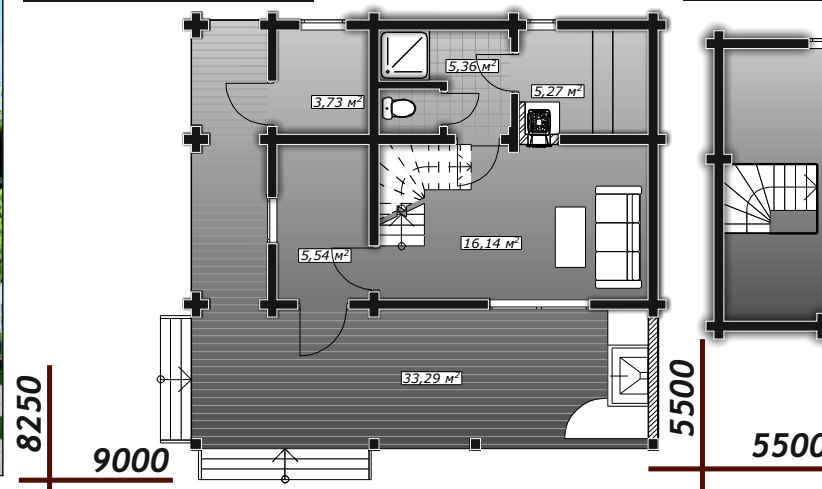
План 1 этажа
